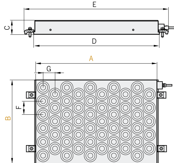
Ausführung B – Polbild versetzt
