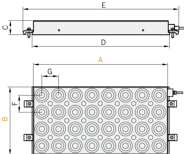
Ausführung A – Polbild linear
